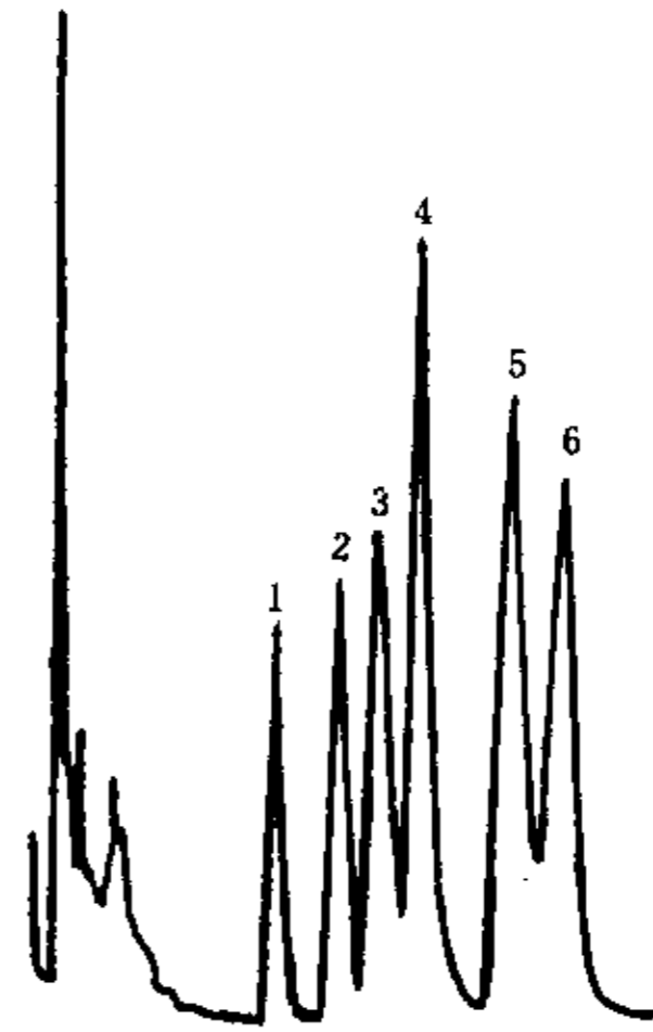
图 2 二硝基苯类化合物气相色谱图
