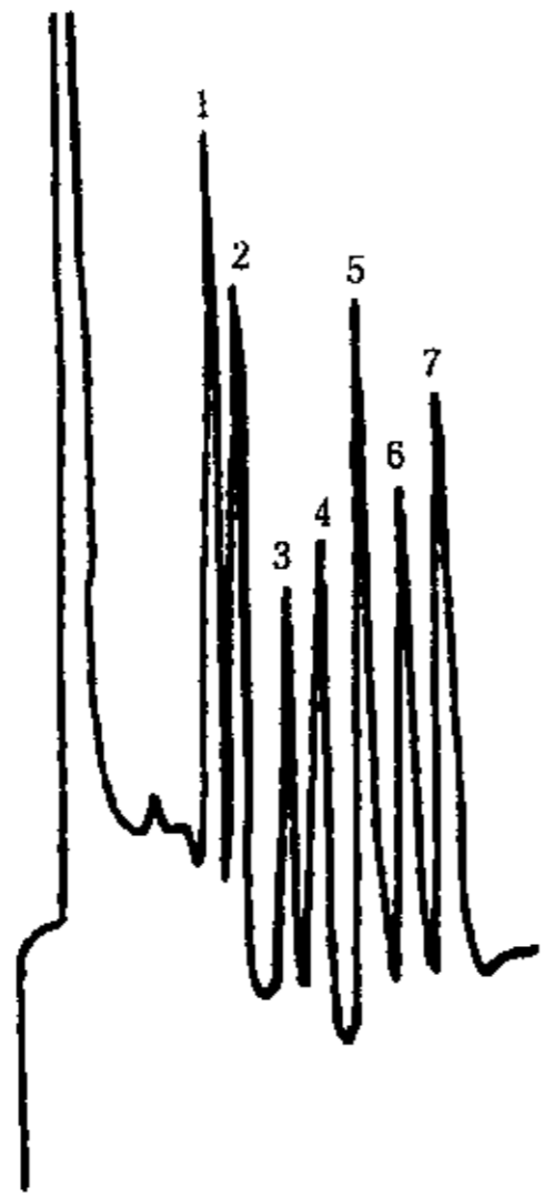
图 1 七种一硝基苯类化合物气相色谱图
